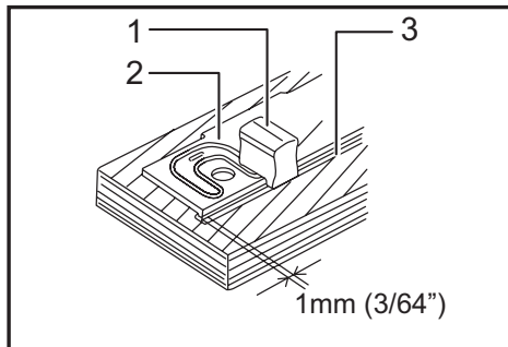
► 1. Support magnétique 2. Plaque de fixation 3. Fer
