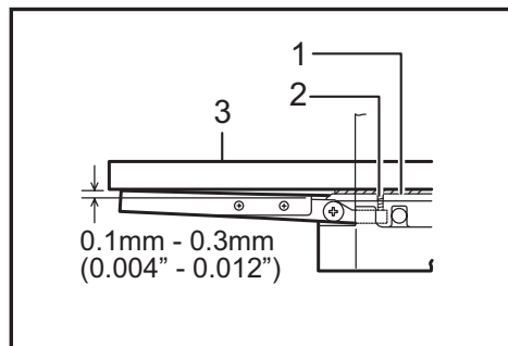
► 1. Tarjeta 2. Tornillo de ajuste 3. Regla
