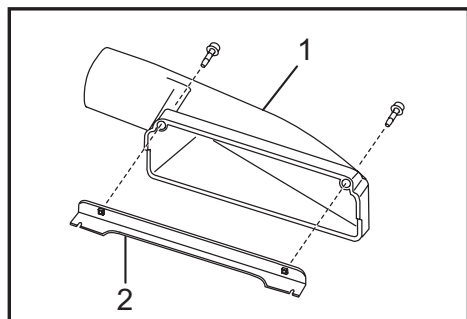
► 1. Carcasa 2. Sujetador de la carcasa
