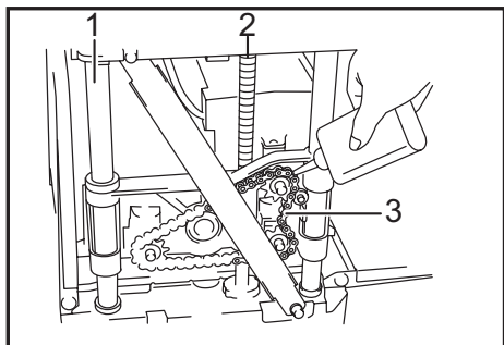
► 1. Columna 2. Tornillo 3. Cadena
