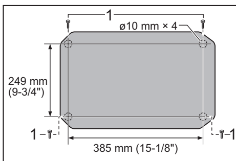
► 1. Perno o tornillo
