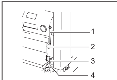
► 1. Butoir 2. Bouton de blocage 3. Poignée de la butée 4. Surface de la table
