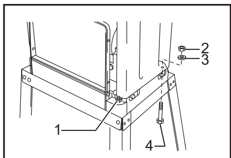
► 1. Tornillo hexagonal 2. Tuerca hexagonal 3. Arandela plana 4. Tornillo hexagonal
