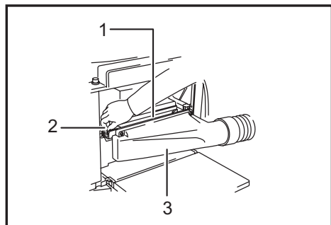
► 1. Protector contra virutas 2. Tornillo de mariposa 3. Carcasa
